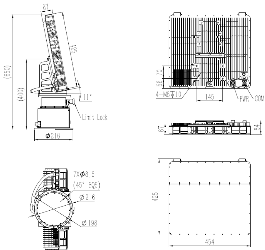
CR-FK02 dimensions structurelles et d'installation (unité : mm)
