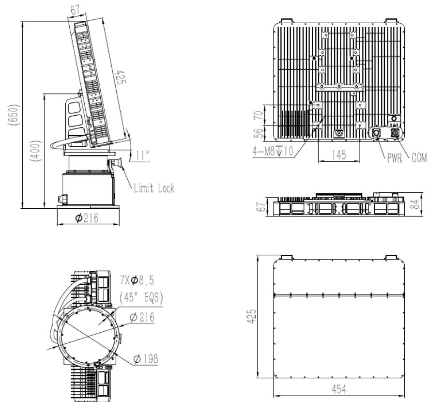
CR-FK02 结构及安装尺寸图 (单位: mm)
