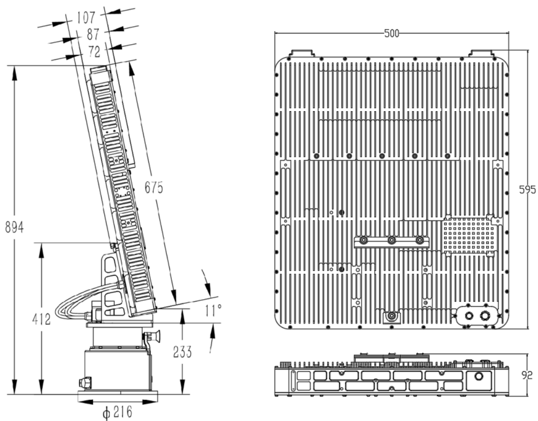
CR-FX10 габаритные и установочные размеры (единица: мм)
