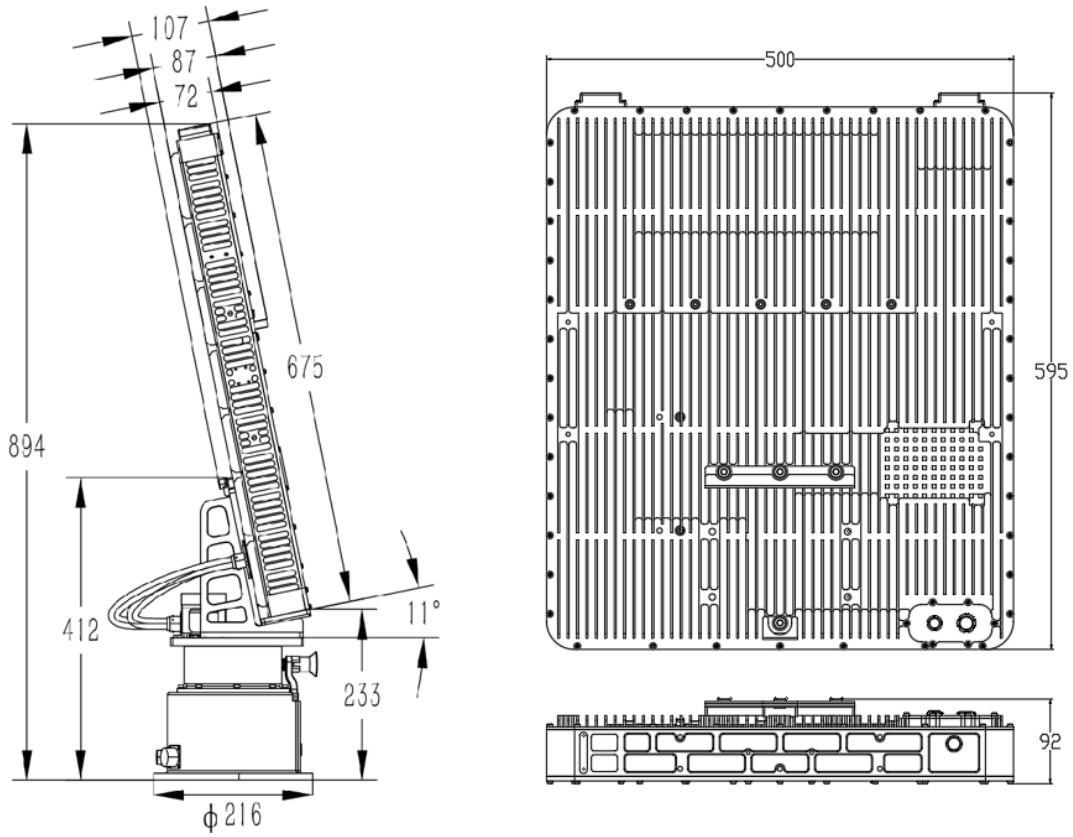
الأبعاد الهيكلية وأبعاد التركيب (الوحدة: مم) CR-FX10
