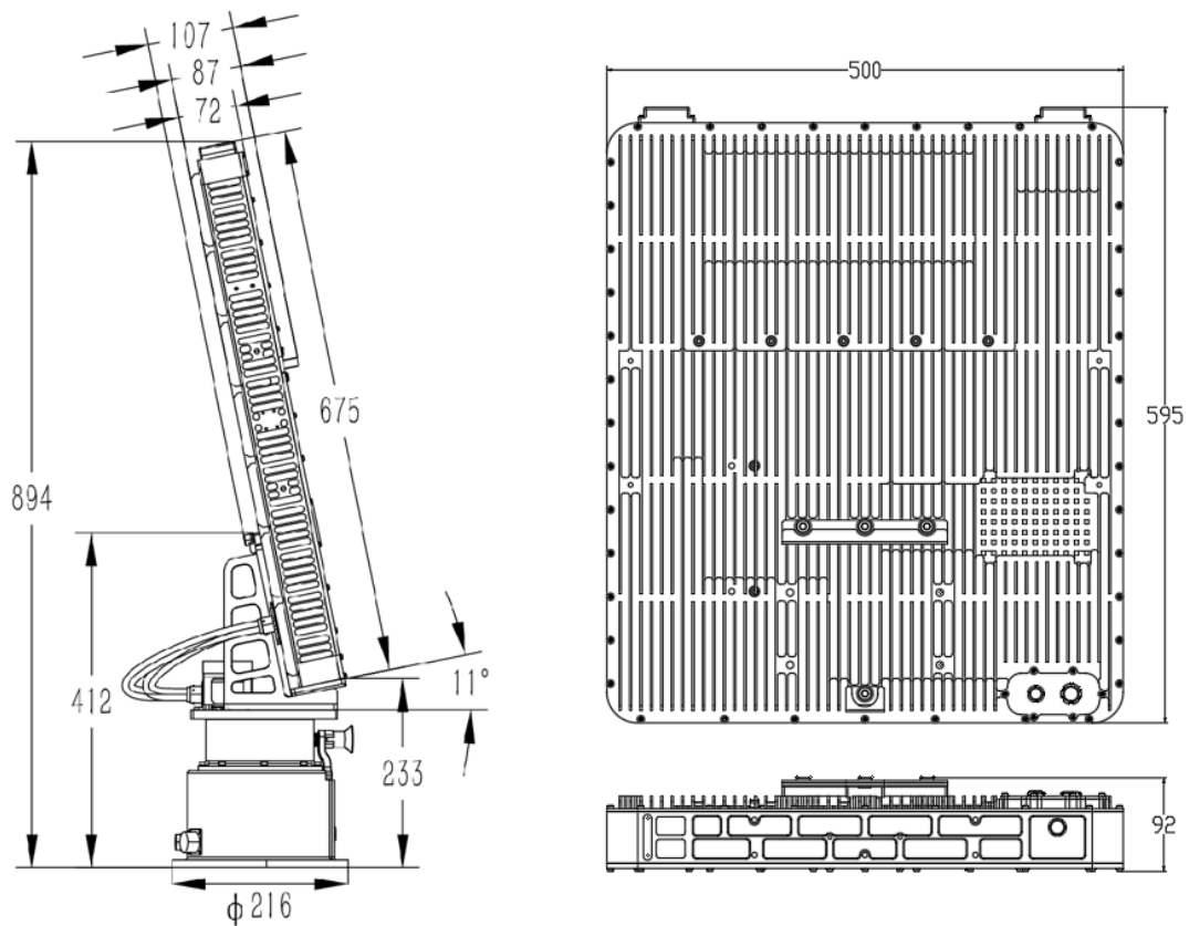
CR-FX10 结构及安装尺寸图 (单位: mm)
