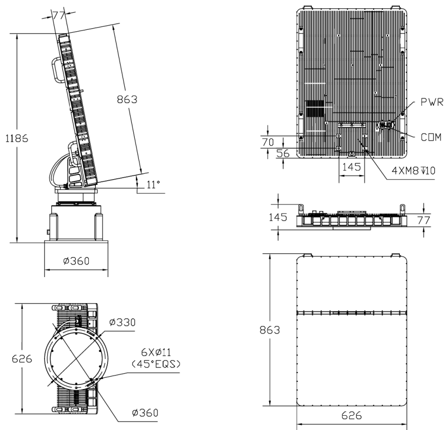
CR-FX18 габаритные и установочные размеры (единица: мм)
