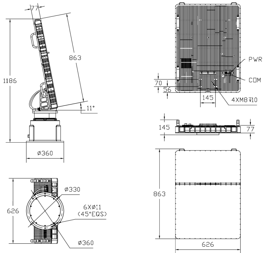
CR-FX18 dimensiones estructurales y de instalación (unidad: mm)
