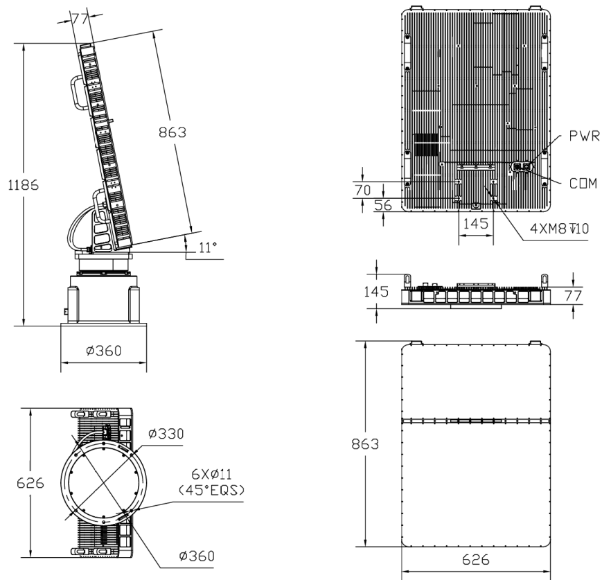
CR-FX18 结构及安装尺寸图 (单位: mm)
