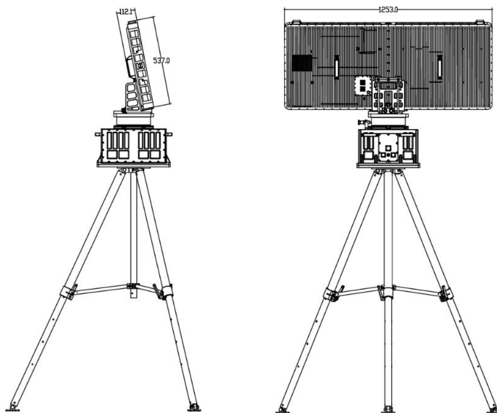
CR-FX20 габаритные и установочные размеры (единица: мм)
