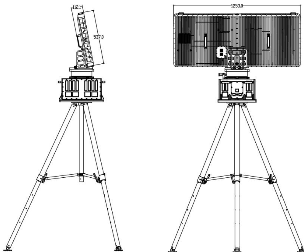
CR-FX20 dimensions structurelles et d'installation (unité : mm)
