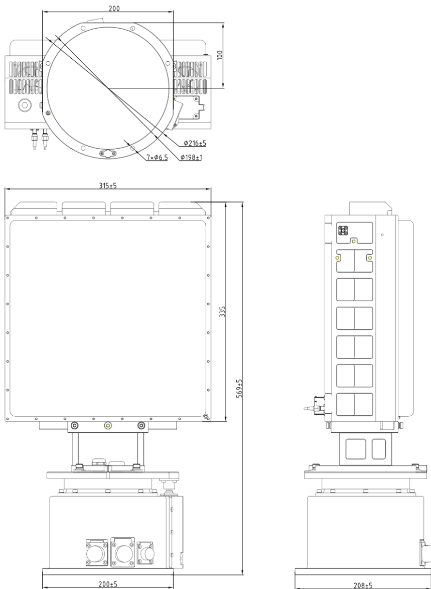
CR-PK05B dimensiones estructurales y de instalación (unidad: mm)
