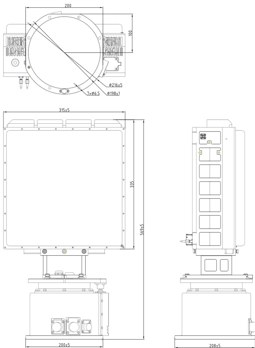
CR-PK05B 结构及安装尺寸图 (单位: mm)
