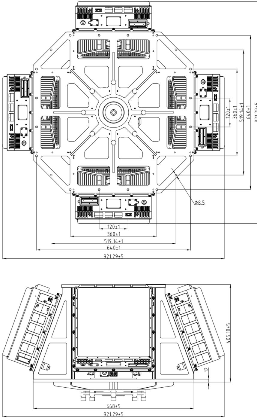
الأبعاد الهيكلية وأبعاد التركيب (الوحدة: مم) CR-PK05C
