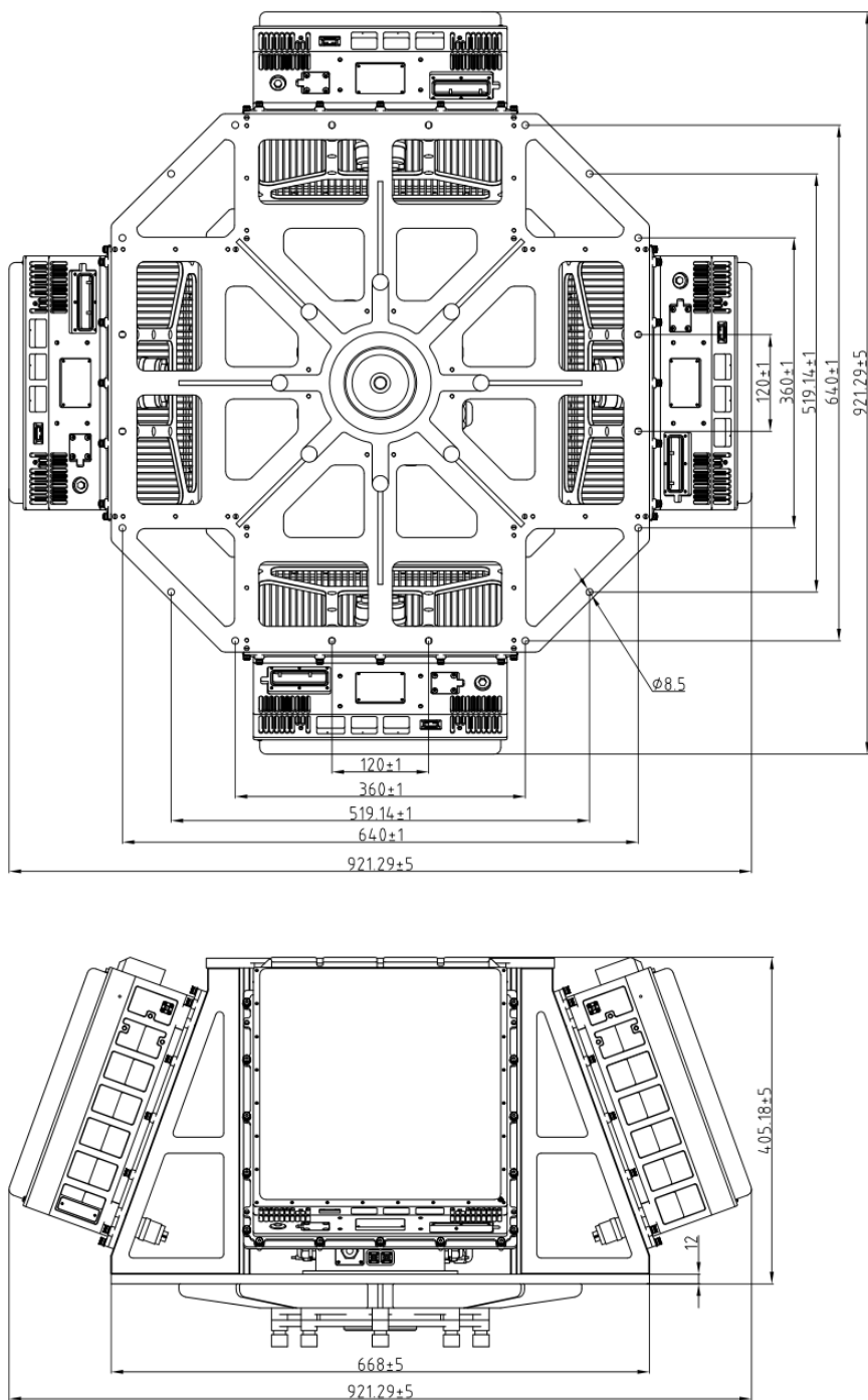
CR-PK05C dimensiones estructurales y de instalación (unidad: mm)
