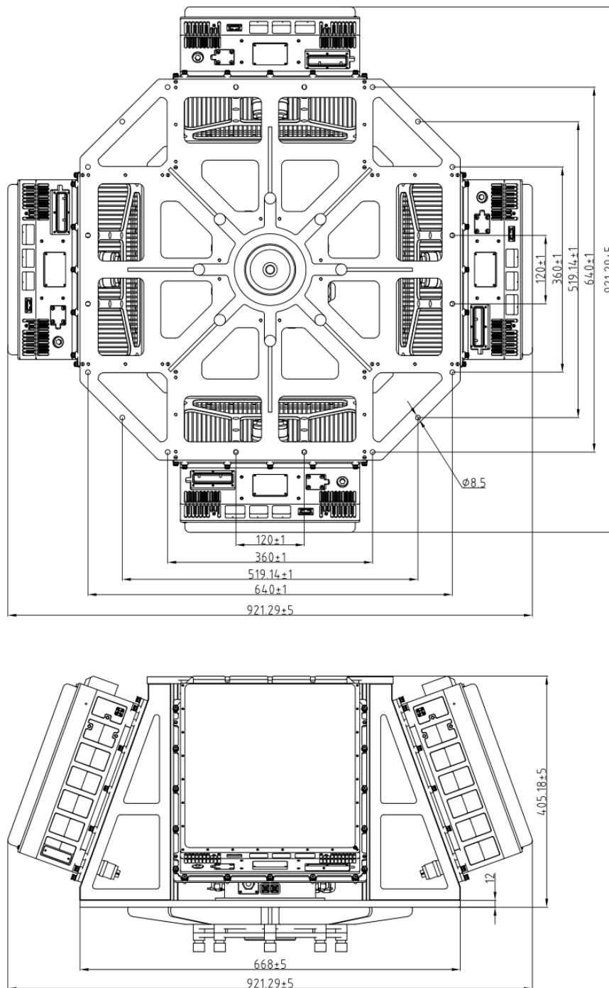
CR-PK05C 结构及安装尺寸图 (单位: mm)
