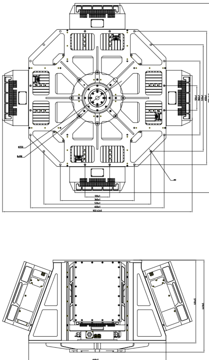
CR-PK13C габаритные и установочные размеры (единица: мм)
