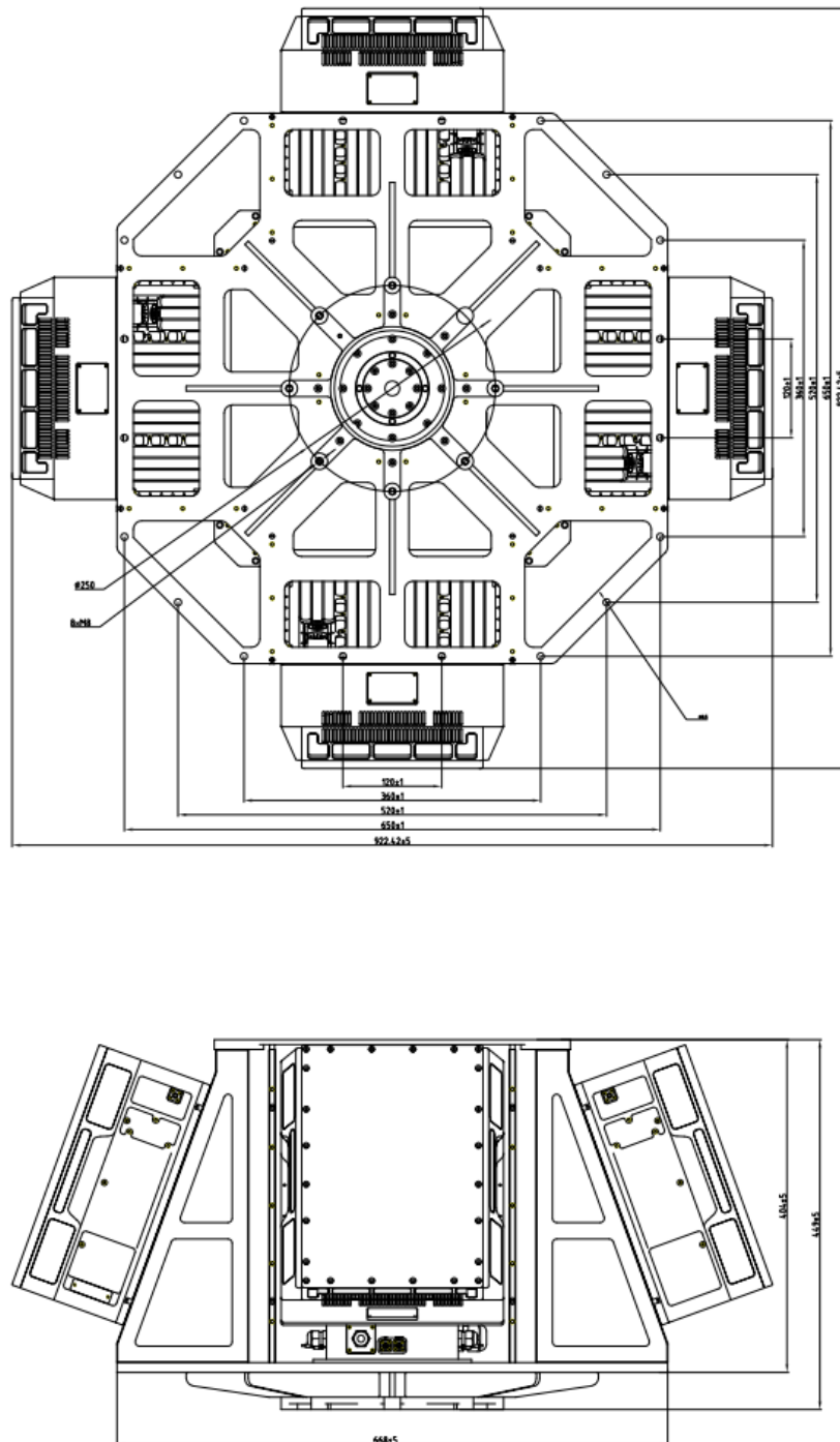
CR-PK13C 结构及安装尺寸图 (单位: mm)
