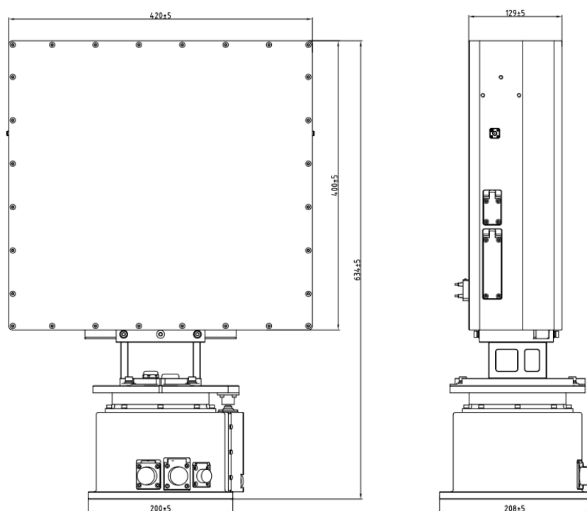
CR-PK14B dimensiones estructurales y de instalación (unidad: mm)
