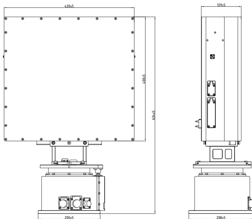
CR-PK14B 结构及安装尺寸图 (单位: mm)
