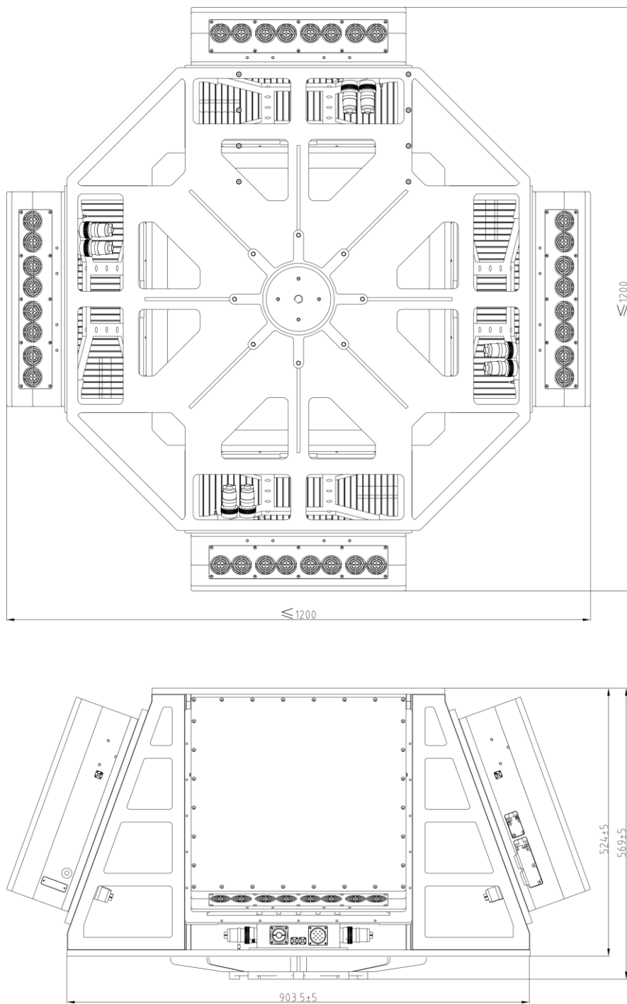
CR-PK14C габаритные и установочные размеры (единица: мм)
