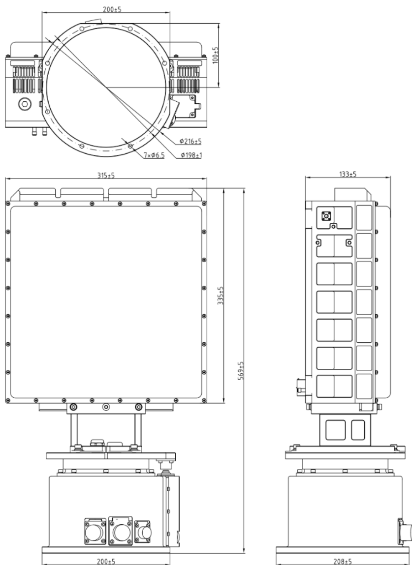
الأبعاد الهيكلية وأبعاد التركيب (الوحدة: مم) CR-PX07B
