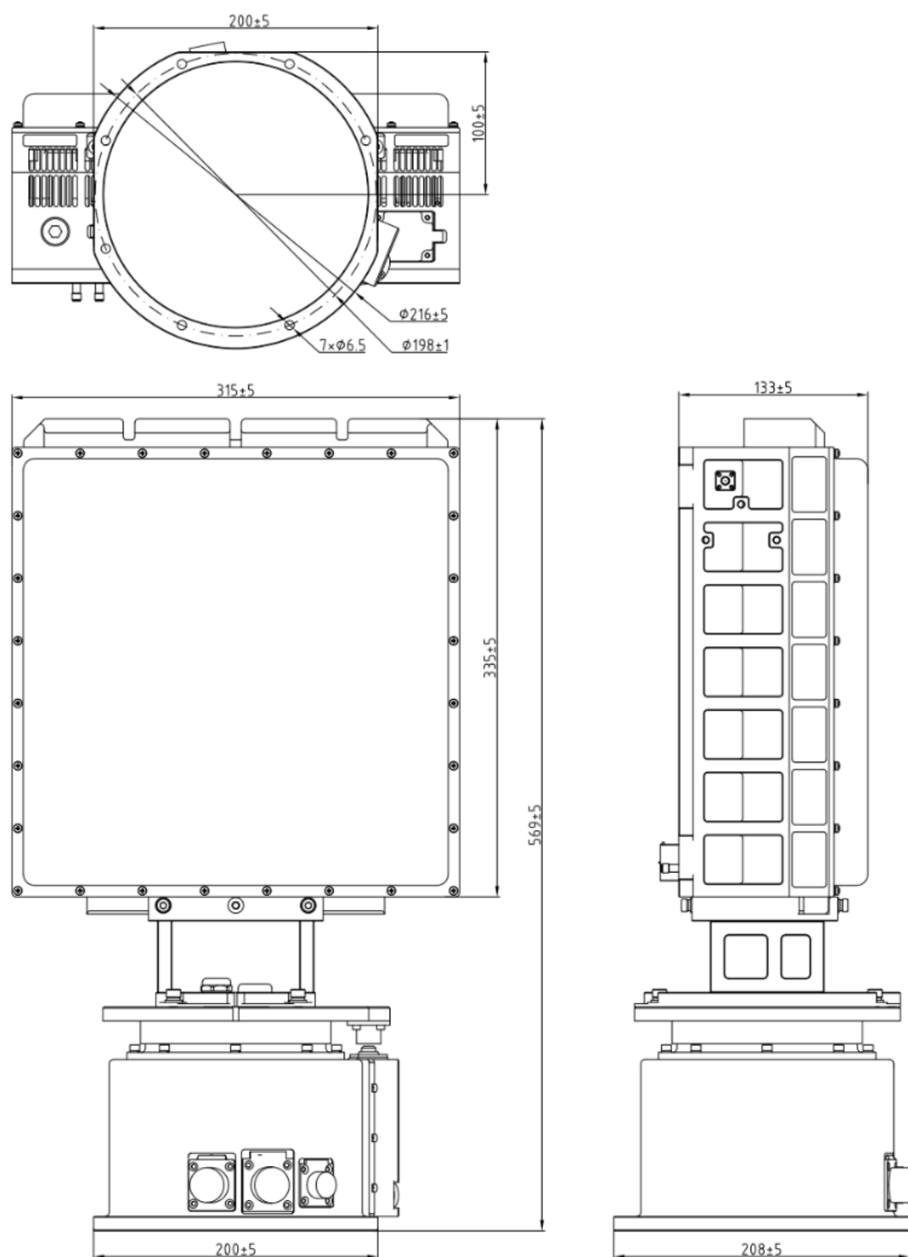
CR-PX07B dimensions structurelles et d'installation (unité : mm)
