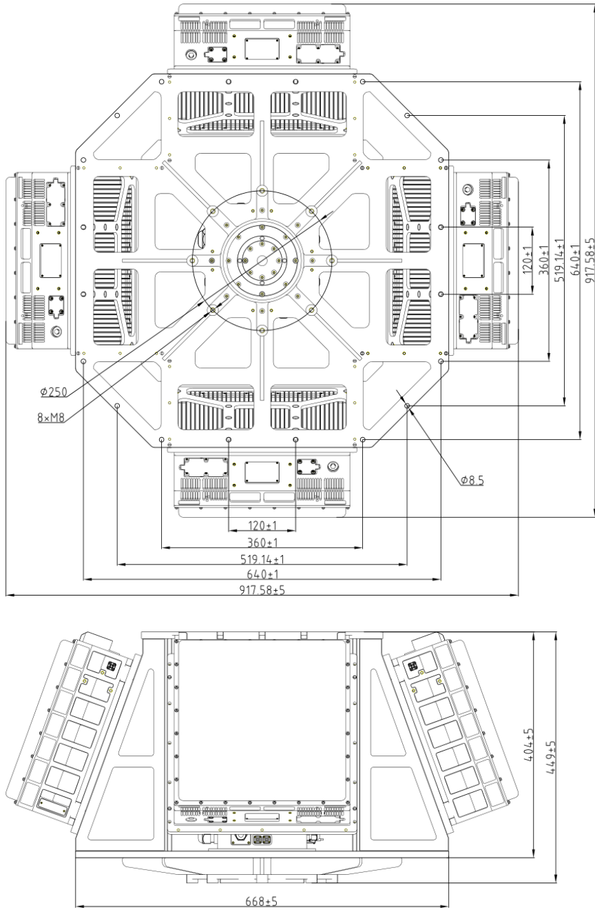
الأبعاد الهيكلية وأبعاد التركيب (الوحدة: مم) CR-PX07C
