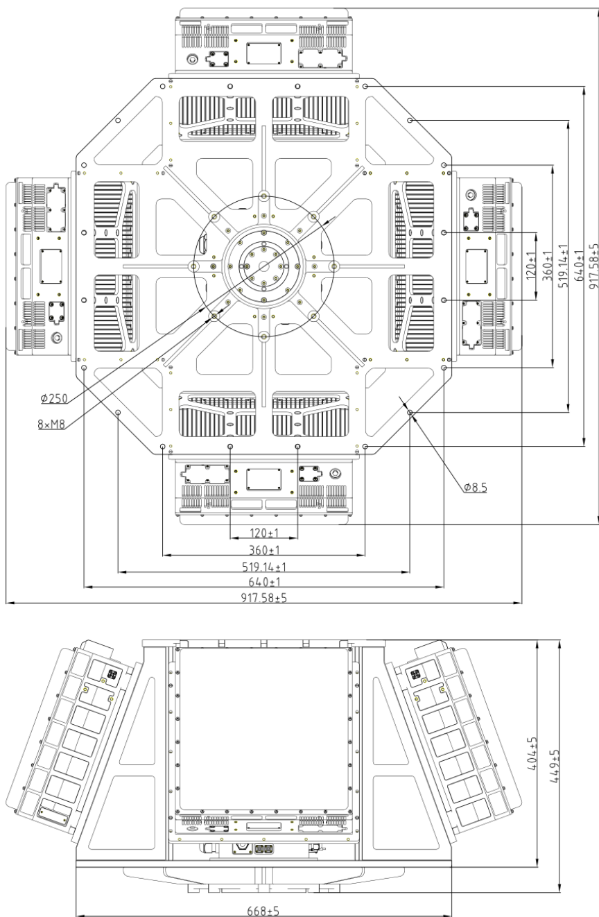
CR-PX07C dimensions structurelles et d'installation (unité : mm)
