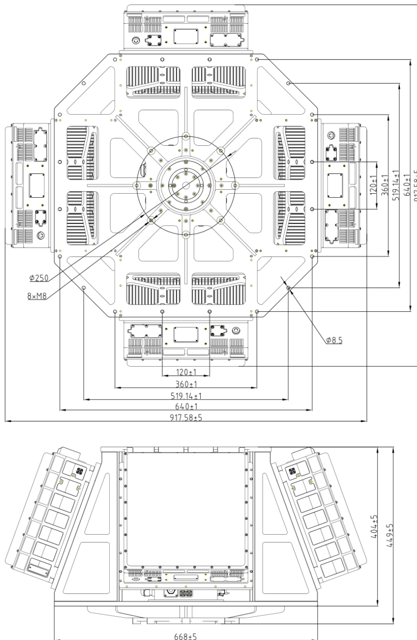
CR-PX07C 结构及安装尺寸图 (单位: mm)
