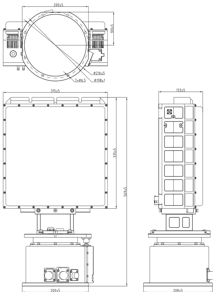
CR-PX08B габаритные и установочные размеры (единица: мм)
