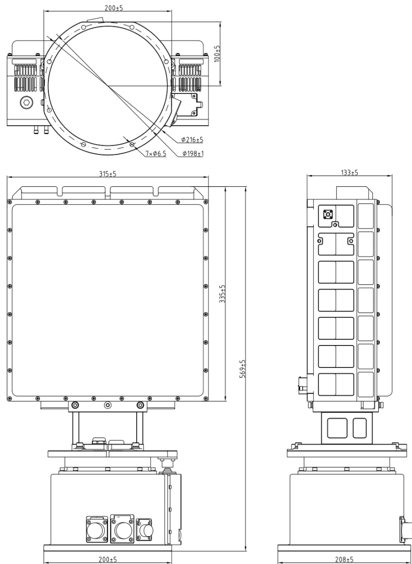
CR-PX08B 结构及安装尺寸图 (单位: mm)
