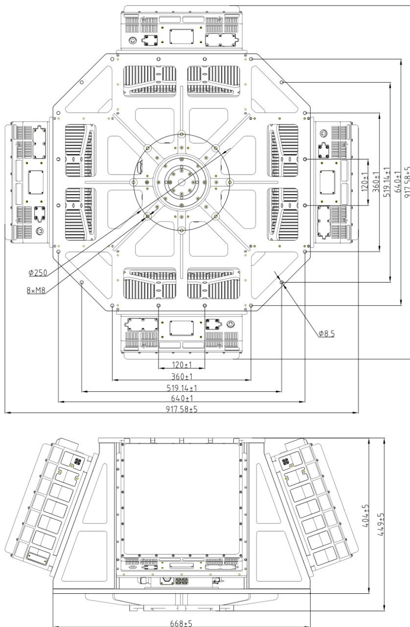
CR-PX08C габаритные и установочные размеры (единица: мм)
