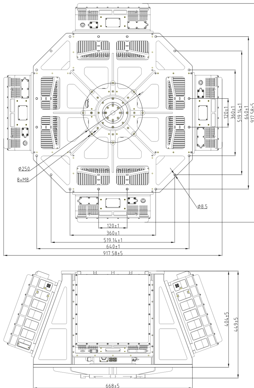
CR-PX08C dimensiones estructurales y de instalación (unidad: mm)
