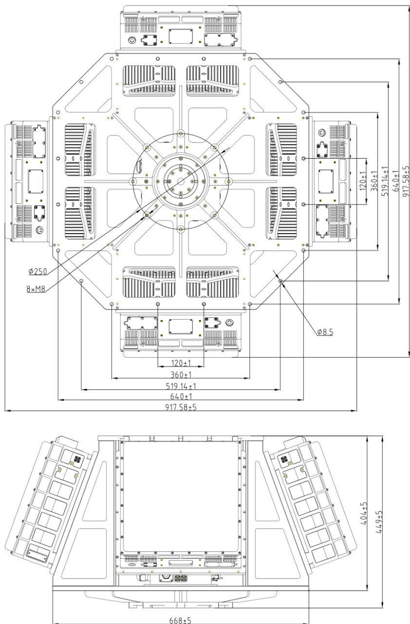
CR-PX08C dimensions structurelles et d'installation (unité : mm)
