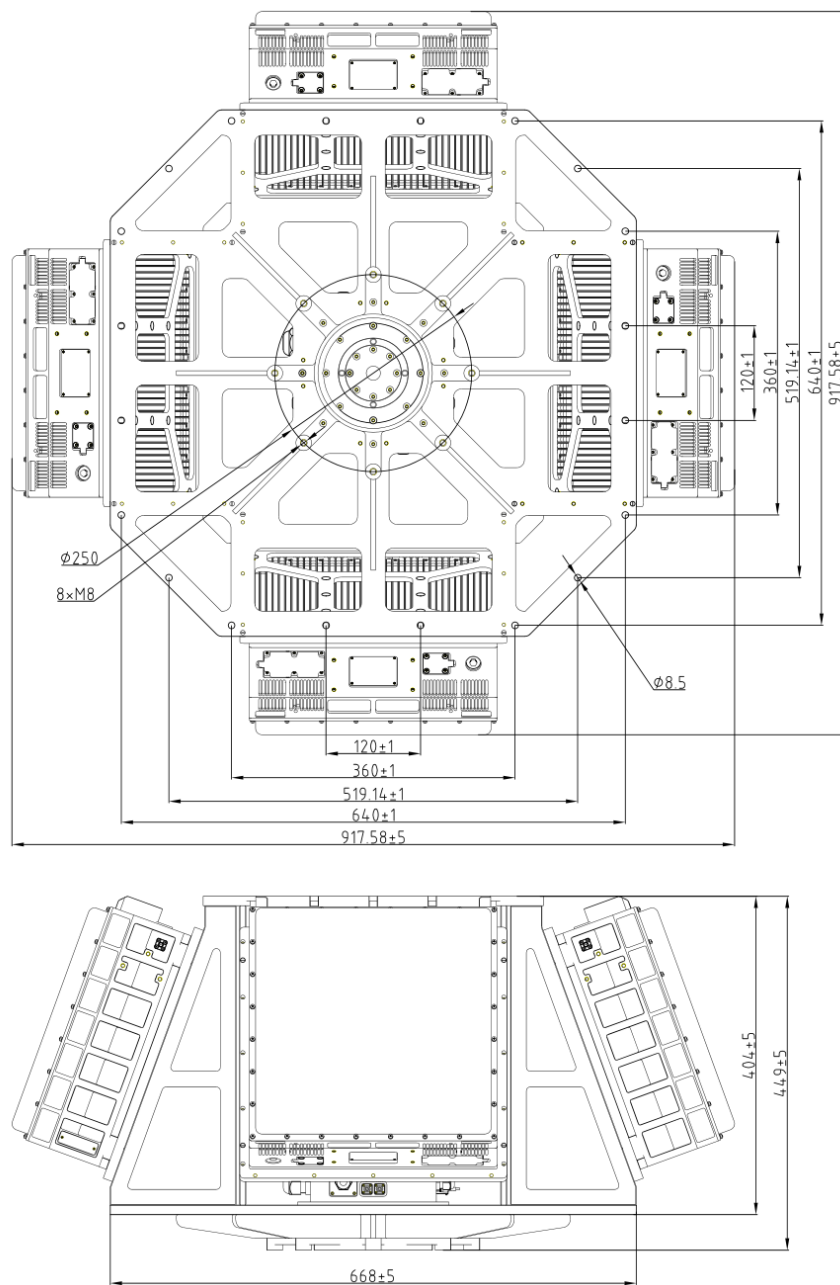
CR-PX08C 结构及安装尺寸图 (单位: mm)
