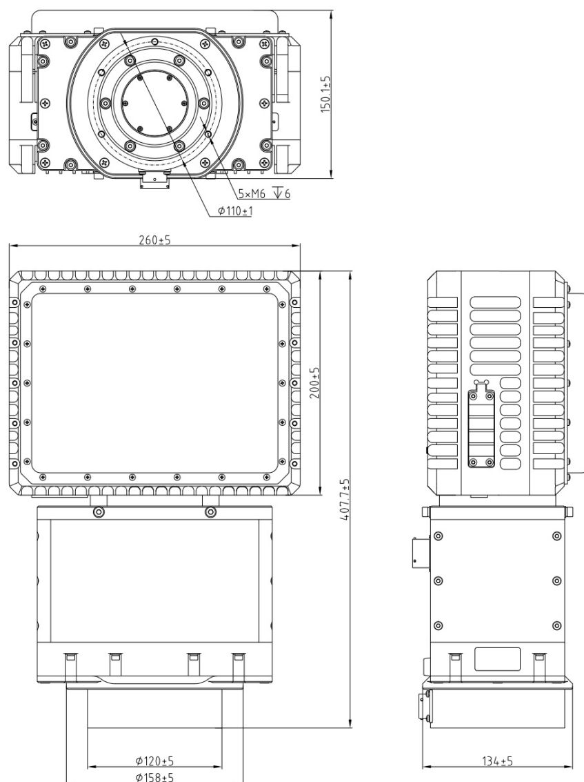
CR-PX10B габаритные и установочные размеры (единица: мм)
