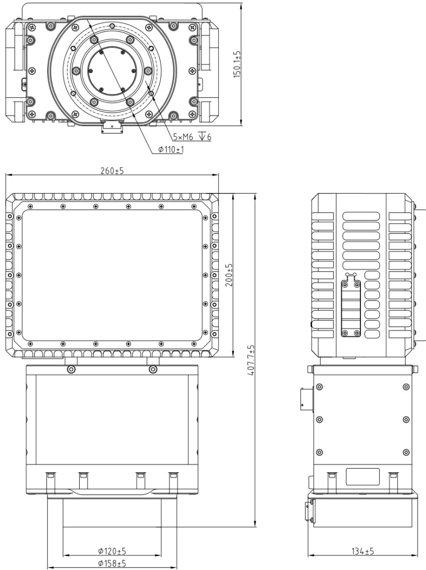
الأبعاد الهيكلية وأبعاد التركيب (الوحدة: مم) CR-PX10B
