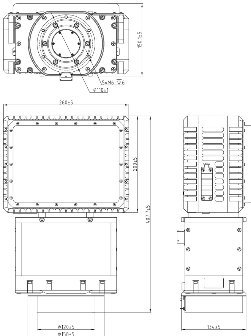
CR-PX10B dimensiones estructurales y de instalación (unidad: mm)
