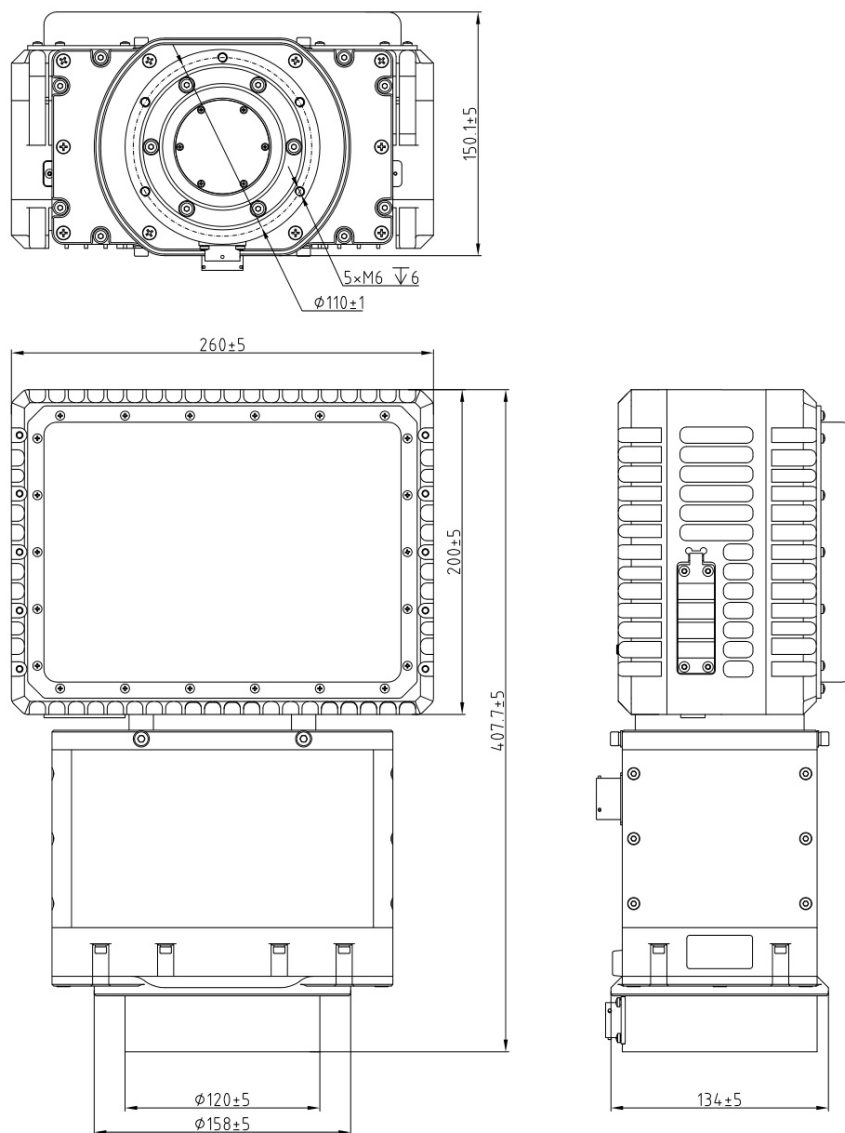
CR-PX10B dimensions structurelles et d'installation (unité : mm)
