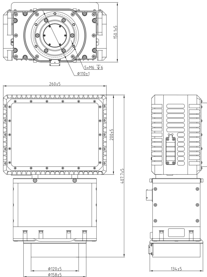
CR-PX10B 结构及安装尺寸图 (单位: mm)
