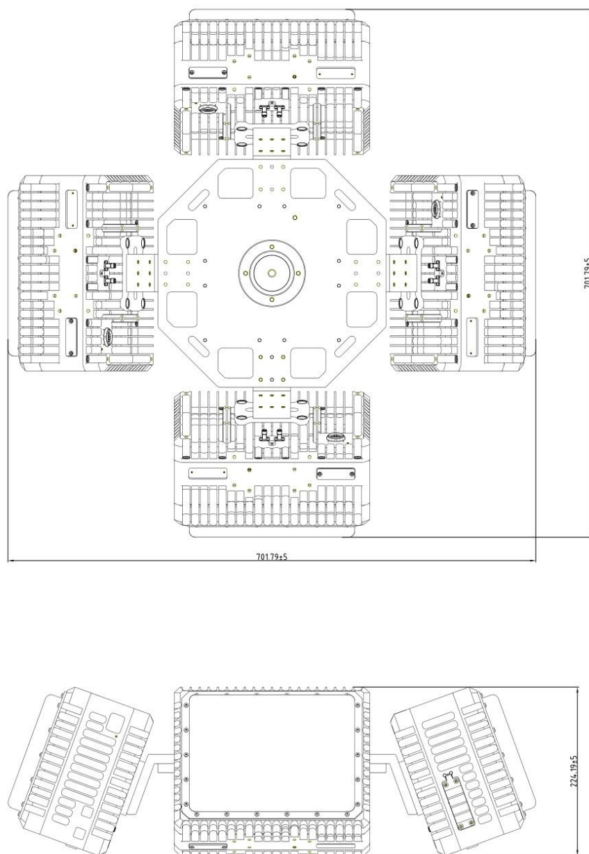
CR-PX10C габаритные и установочные размеры (единица: мм)
