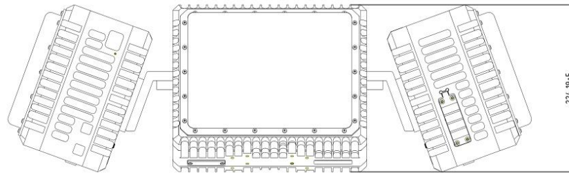
الأبعاد الهيكلية وأبعاد التركيب (الوحدة: مم) CR-PX10C
