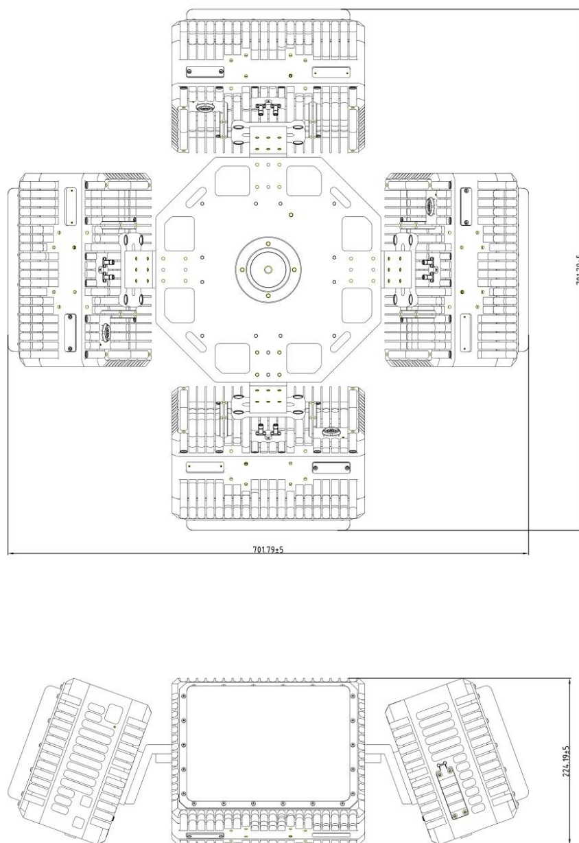
CR-PX10C dimensiones estructurales y de instalación (unidad: mm)
