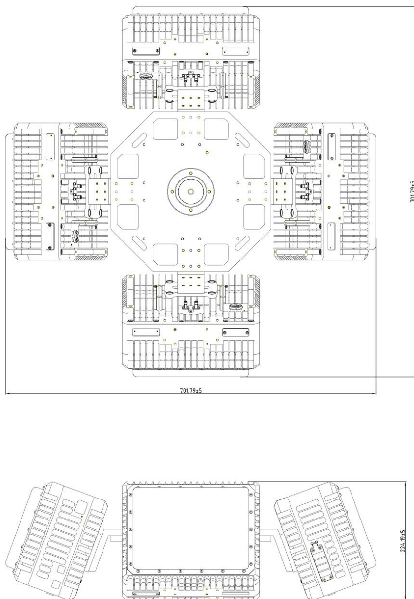
CR-PX10C dimensions structurelles et d'installation (unité : mm)
