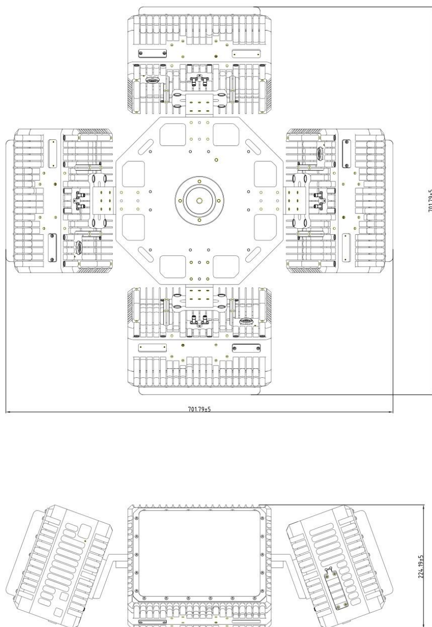
CR-PX10C 结构及安装尺寸图 (单位: mm)
