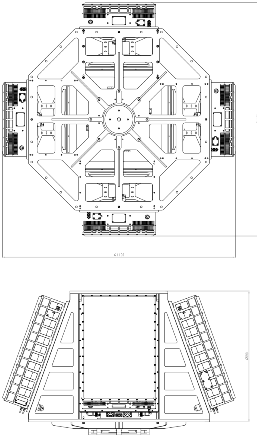
CR-PX11C габаритные и установочные размеры (единица: мм)
