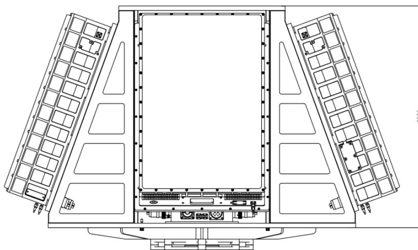
CR-PX11C dimensiones estructurales y de instalación (unidad: mm)
