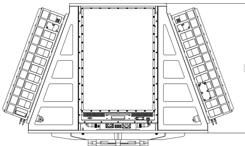
CR-PX11C dimensions structurelles et d'installation (unité : mm)
