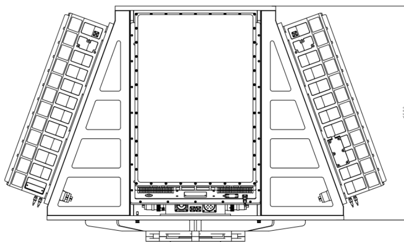
CR-PX11C 结构及安装尺寸图 (单位: mm)
