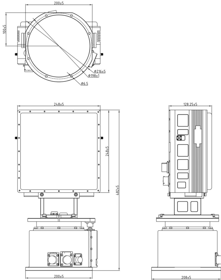
الأبعاد الهيكلية وأبعاد التركيب (الوحدة: مم) CR-PX15B
