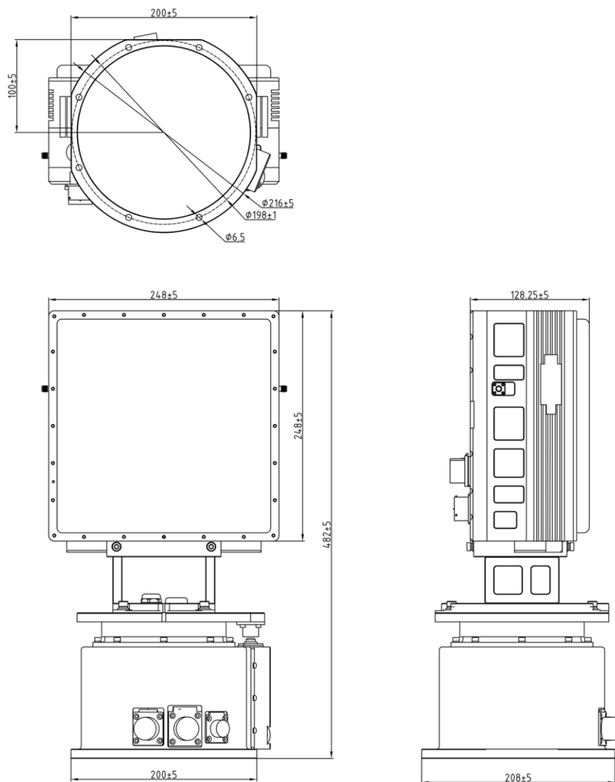
CR-PX15B dimensions structurelles et d'installation (unité : mm)
