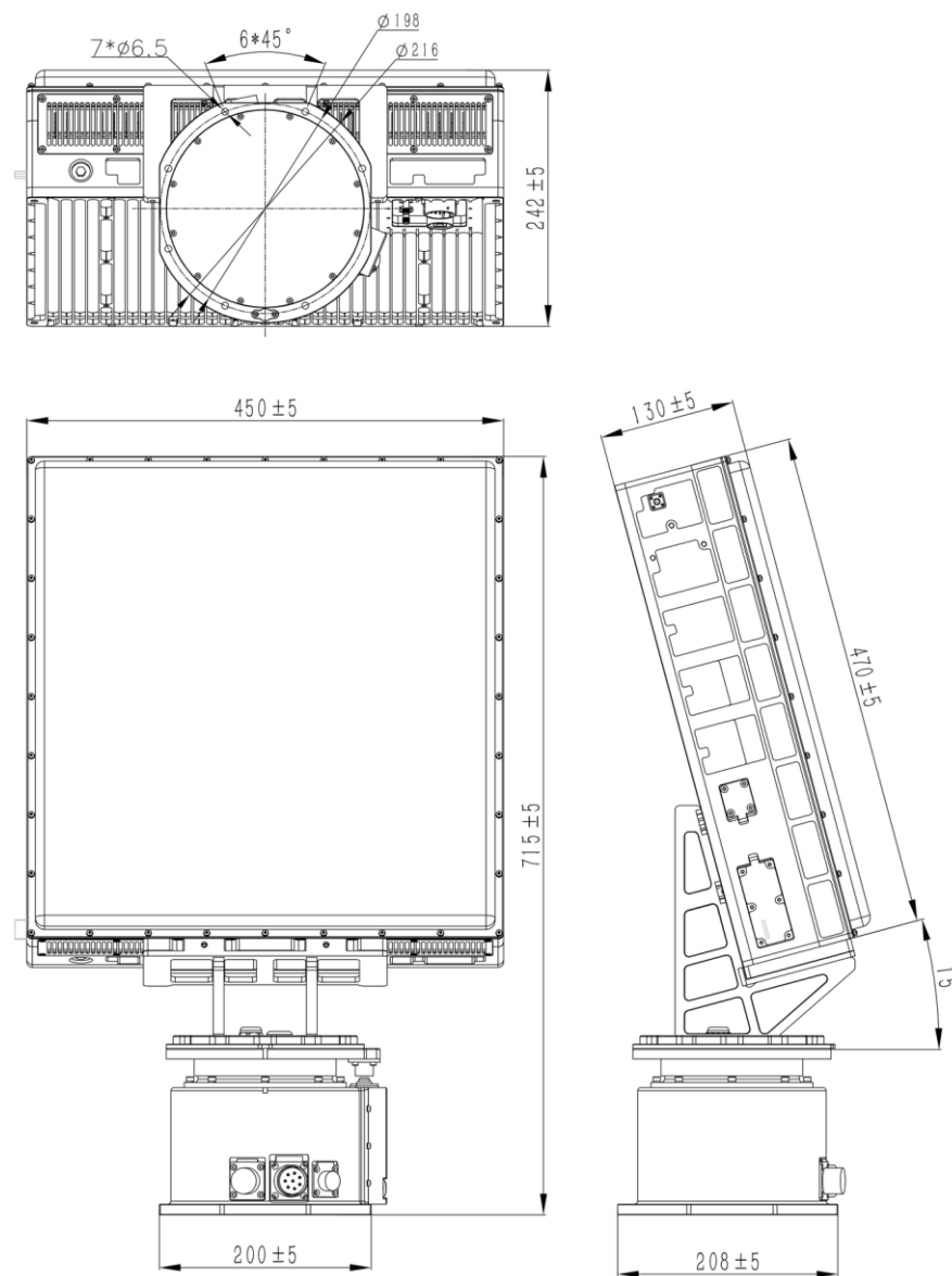
CR-PX16B 结构及安装尺寸图 (单位: mm)
