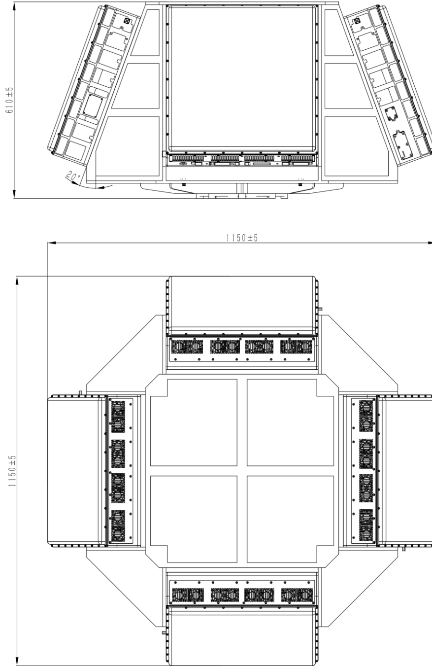
الأبعاد الهيكلية وأبعاد التركيب (الوحدة: مم) CR-PX16C
