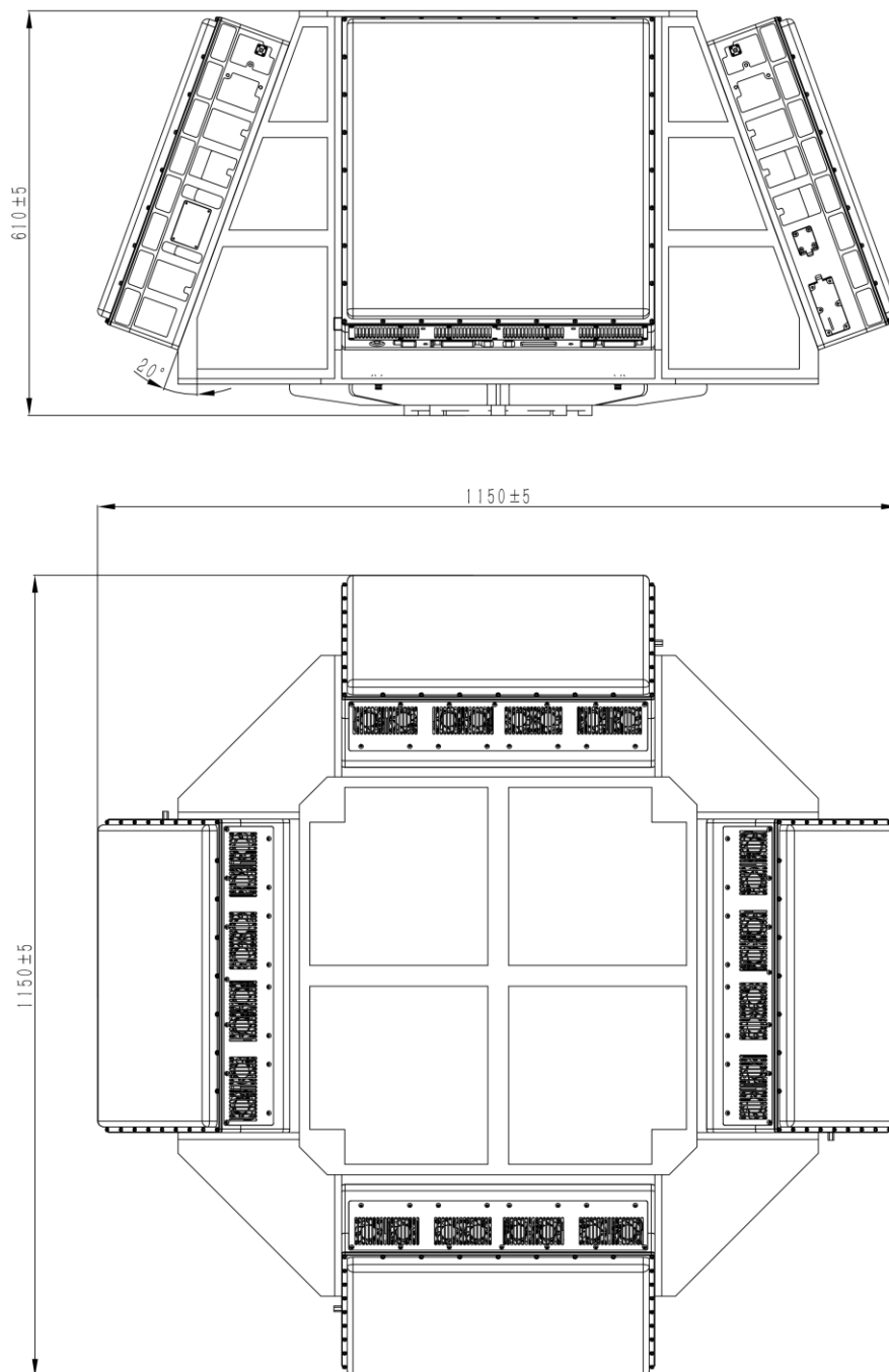
CR-PX16C dimensiones estructurales y de instalación (unidad: mm)
